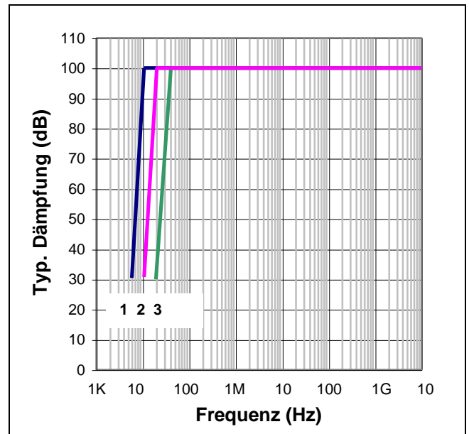
Einfügungs-Dämpfung nach CISPR 17 in 50 Ω-Systemen, asymmetrisch, mit und ohne Last
